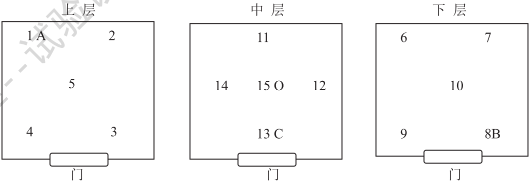
图 2 设备容积大于 2\text{m}^3 布点示意图
