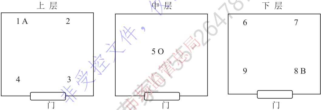
图 1 设备容积小于等于 2\text{m}^3 布点示意图
